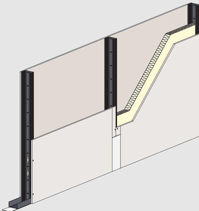
Beispiel: einlagige Beplankung
