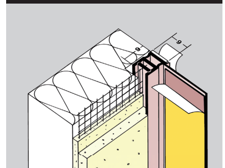
Laibungsanschlussprofil 3728 WDVS
