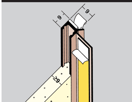
Laibungsanschlussprofil 3712 Innenputz
