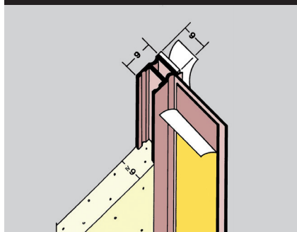
Laibungsanschlussprofil 3726 Außenputz
